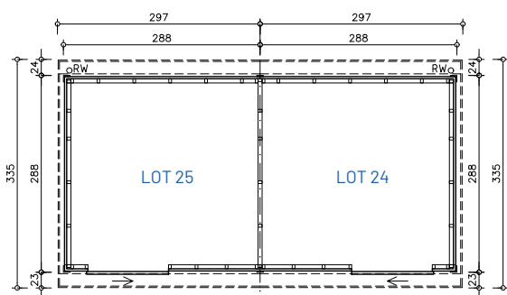
GELIJKVLOERS
