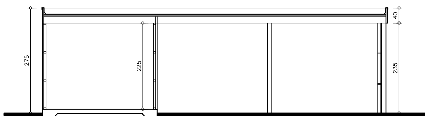
DOORSNEDE
