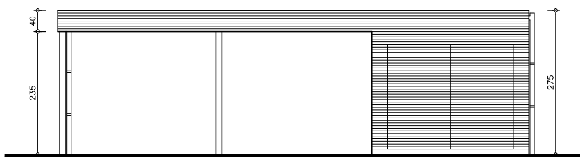
ZIJGEVEL RECHTS
