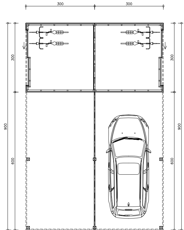
GRONDPLAN
