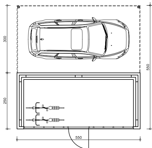
Grondplan
