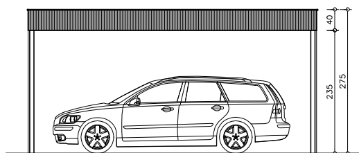
Achtergevel
