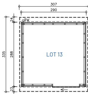
GELIJKVLOERS
