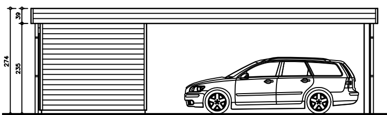
CARPORT Woning 3 & 5 ZIJGEVEL LINKS
