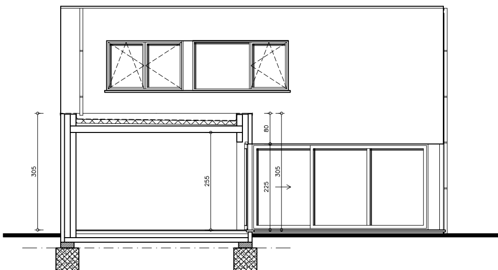
LOT J12 ACHTERGEVEL
