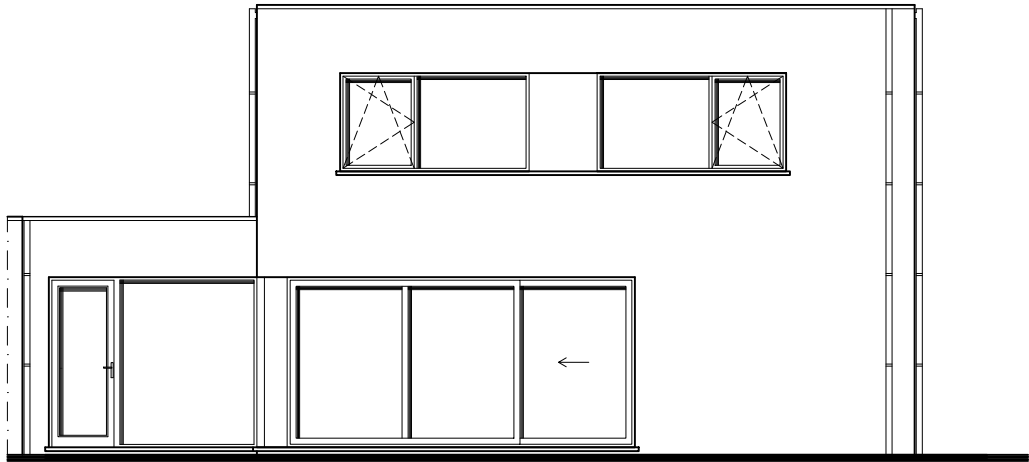
LOT J12 ZIJGEVEL LINKS
