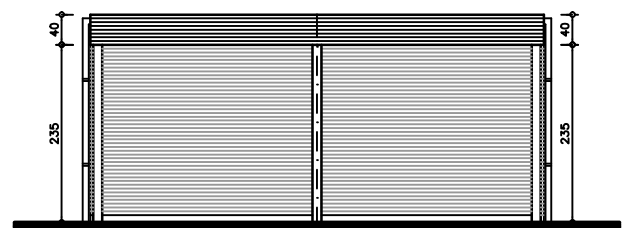
Voorgevel
