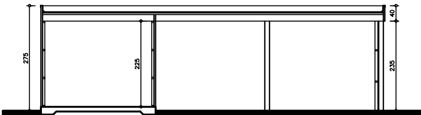
Doorsnede
