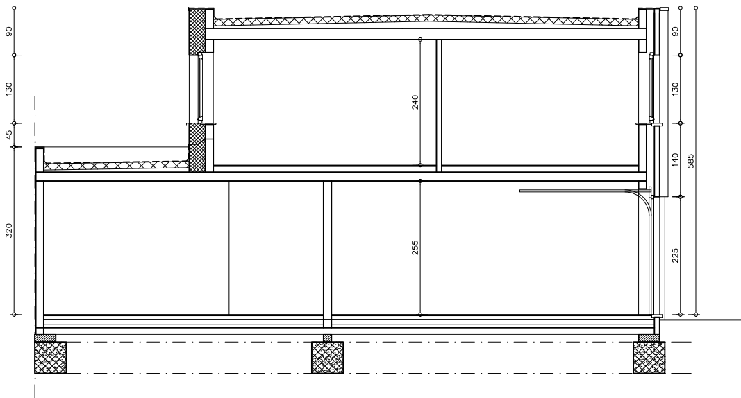
DOORSNEDE
